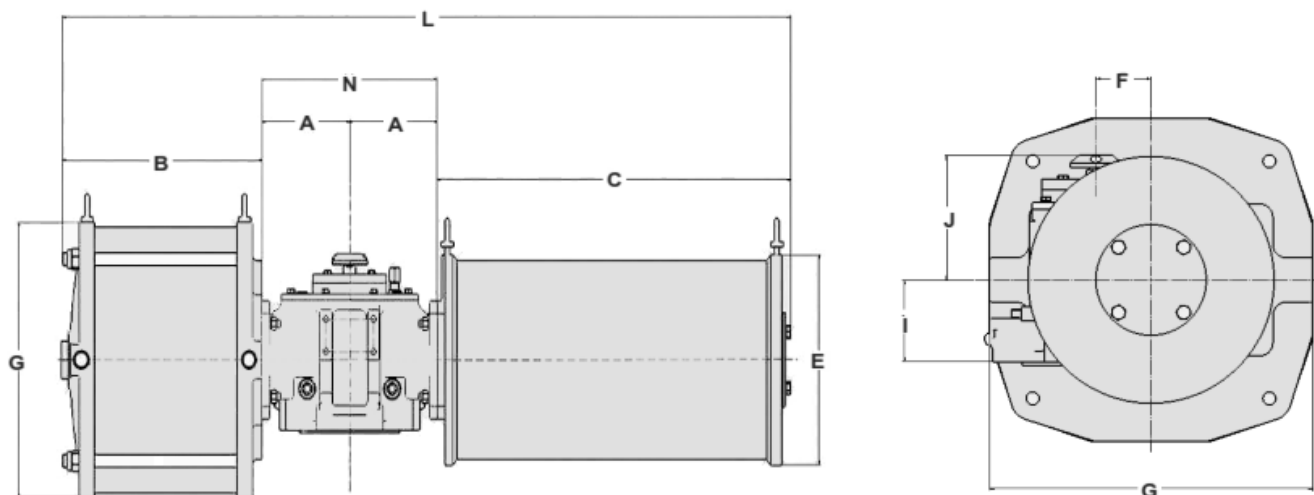
RozmĚry (mm)
