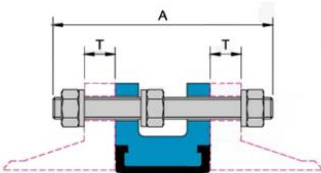
Flanschtyp DN500
