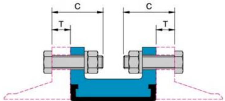
Flanschtyp DN600-DN900
