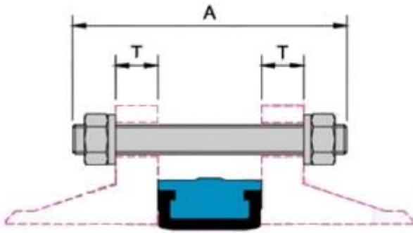
Zwischenflanschgehäuse DN40-DN900
