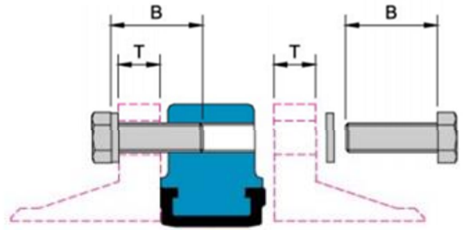
Anflanschgehäuse DN40-DN600
